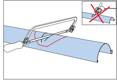
Fémfűrészsel készítsük el a kivágást az ereszcsonornában (flex használata tilos!).
