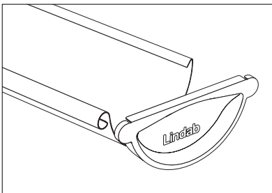
Az RG öntömítő véglemezt illesszük a csatorna végére bepattintással.
