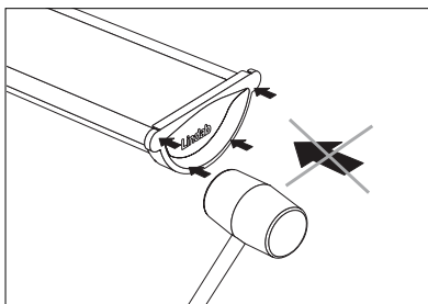
Végül az RG véglemezt műanyag kalapáccsal rögzítjük az ereszcsonorna végére.
