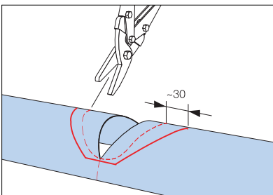
Ollóval fejezzük be mindkét oldalt a kivágást, az ábrán látható módon.
