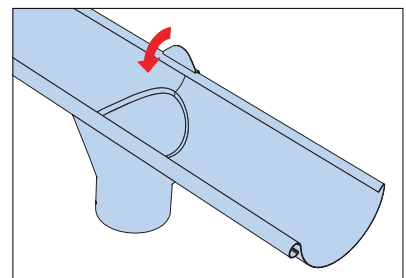
A betorkolócsonkot illesszük rá a kivágásra és pattintsuk rá az ereszcsonornára.
