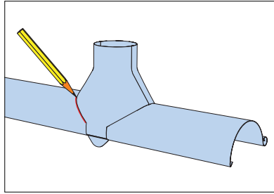
Az ereszcsonornára helyezett betorkolócsonkot használjuk mintának.
