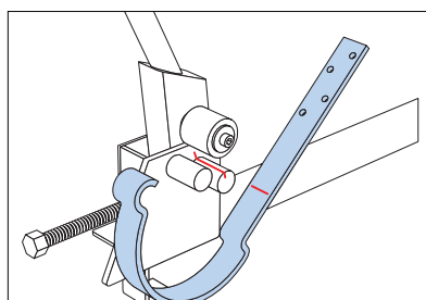
Hajlítsuk meg a csatornatartókat a jelölésnél!
